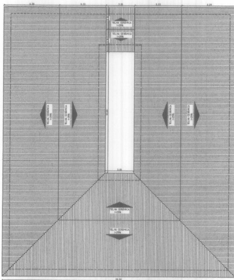
PLANTA DE COBERTURA esc 1:125
